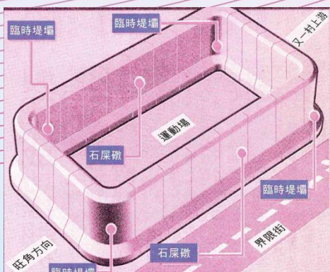
本會向渠務署建議大坑東興建大型蓄洪池以解決九龍西區水浸問題
